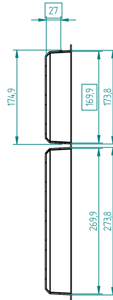
Schnitt A-A
