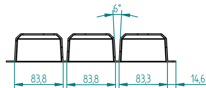
Schnitt B-B
