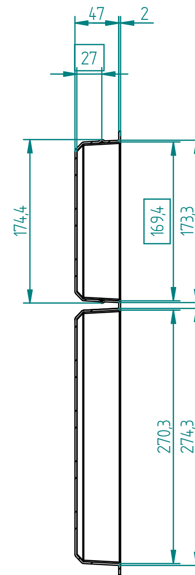
Schnitt A-A
