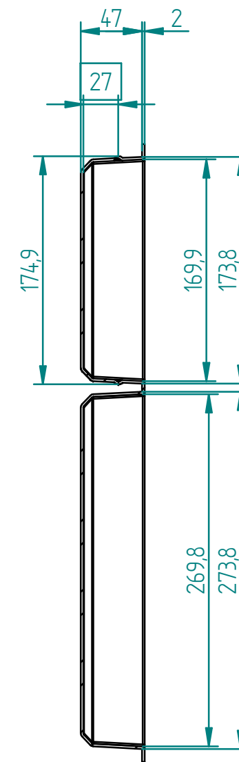
Schnitt A-A
