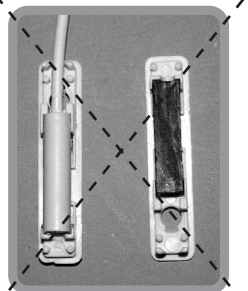
FALSCHE Montage Versetzte Anordnung
