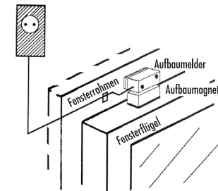
Melder- Halter Befestigung an dem Fensterahmen Magnet- Halter Befestigung an das Fenster
