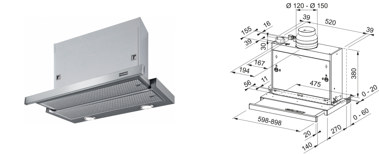
Flachschirmhaube Omnia, FTCO 60 XS 60 cm, Edelstahl, Aktivkohlefilter nicht im Lieferumfang enthalten
