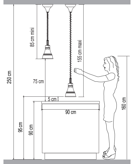
Beispiel für die Installation auf einer Mittelinsel
