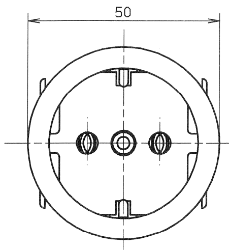
Einbauausschnitt für Rastbefestigung Wanddicke 0,6mm-1,5mm
