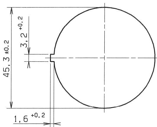
Einbauausschnitt für Rastbefestigung Wanddicke 0,6mm-1,5mm
